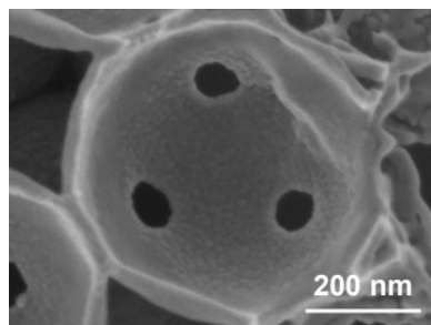
Opale inverse de TiO 2 élaboré par ALD
